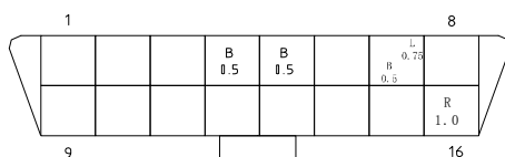
诊断接口
